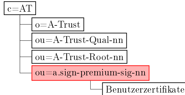
Abbildung 2: A-Trust Verzeichnisbaum
